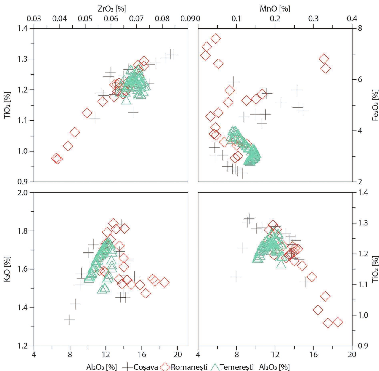
Fig. 19. Bi-plots of different oxides for Românești, Coșava and Temerești.
